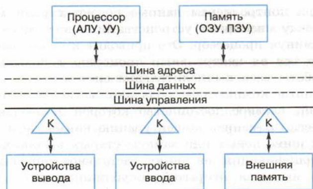
Рис. 2.7. Функциональная схема компьютера (К — контроллер)
