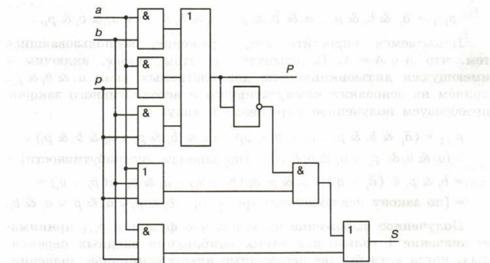
Рис. 4.10. Схема одноразрядного сумматора
