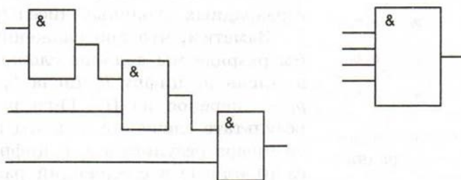
Рис. 4.7. Схема и обозначение четырёхвходового конъюнктора
